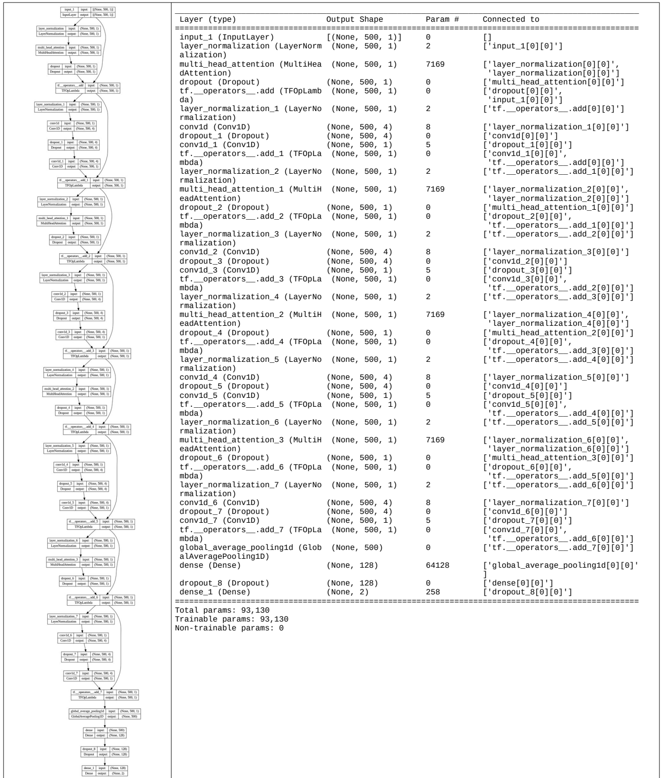
Figura 8: Arquitetura da rede Transformer para classificar FordA.
