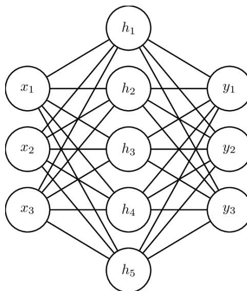
Figura 9: A rede do programa 4 recebe 28×28=784 dados de entrada (x), possui uma camada escondida com 400 neurônios (h) e uma camada de saída (y) com 10 neurônios – esta figura apresenta quantidades bem menores de neurônios.
